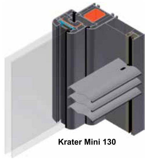
Die Krater Jalousie mit sichtbarer Blende
