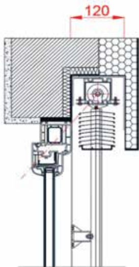
Querschnitt Krgan Unterputz
