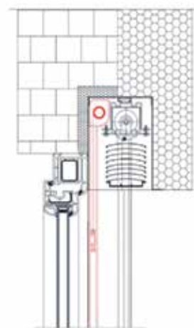
Querschnitt Krgan mit einem Rollo Insektengitter
