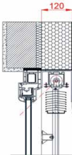
Querschnitt Krgan sichtbare Blende des Jalousiekastens
