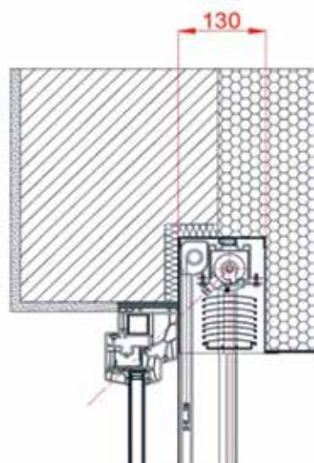
Querschnitt der Krater Mini Jalousie mit Rollo-Insektenschutz
