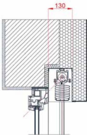
Querschnitt der Krater Mini Jalousie ohne Rollo-Insektenschutz
